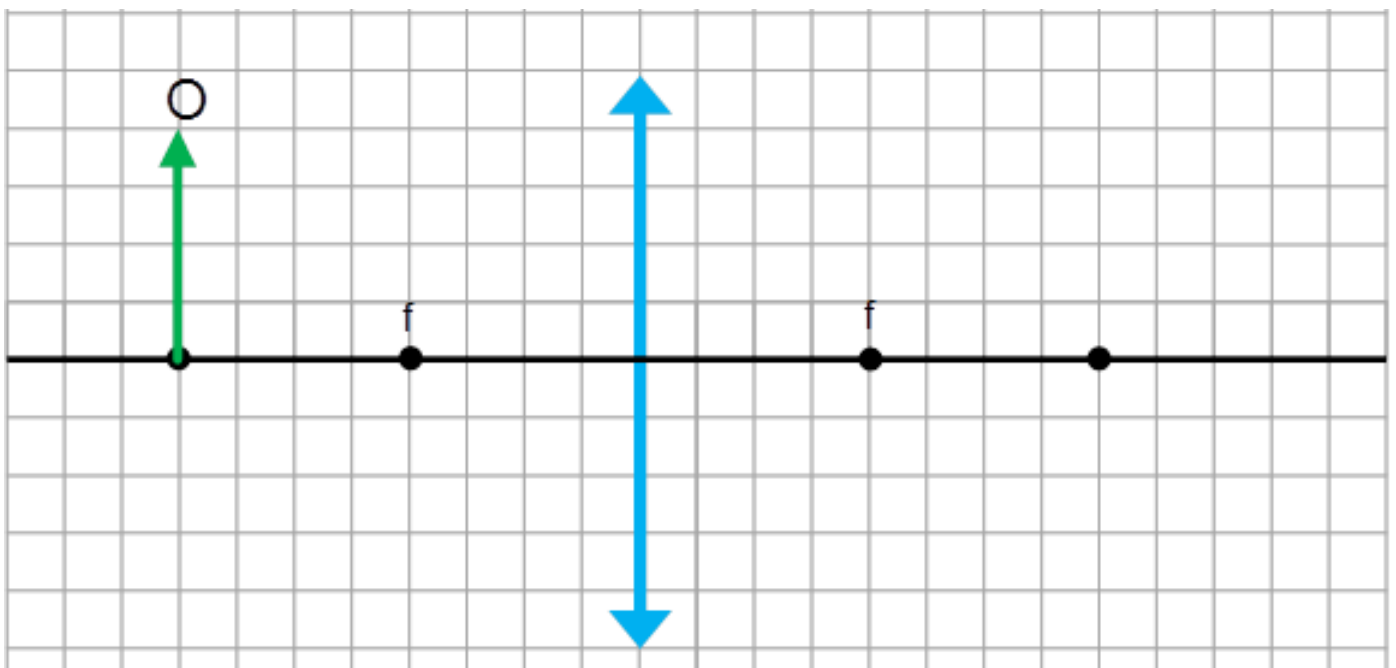
Figura 4: Objeto no anti-principal
