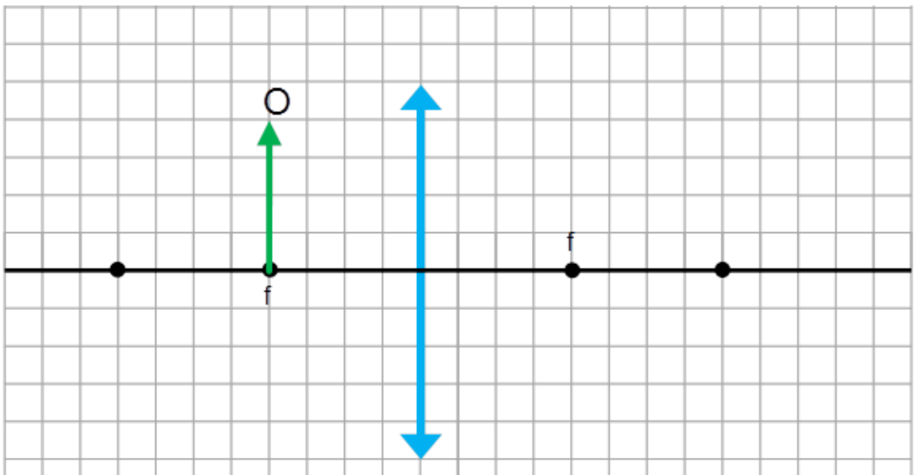
Figura 2: Objeto no foco
